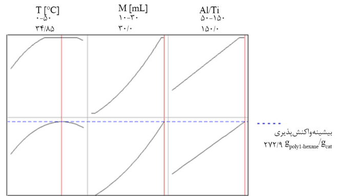
شکل ۴- تعیین مقدار بیشینه واکنش پذیری کاتالیزور در پلیمر شدن ۱-هگزن با استفاده از روش سطح پاسخ.
