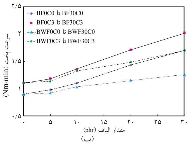
شکل ۳- تغییرات: (الف) زمان پخت و (ب) سرعت پخت آمیزه‌های تهیه شده با ترکیب درصدی مختلف الیاف نو و ضایعاتی برای آمیزه‌های با و بدون نانوخاک‌رس.
